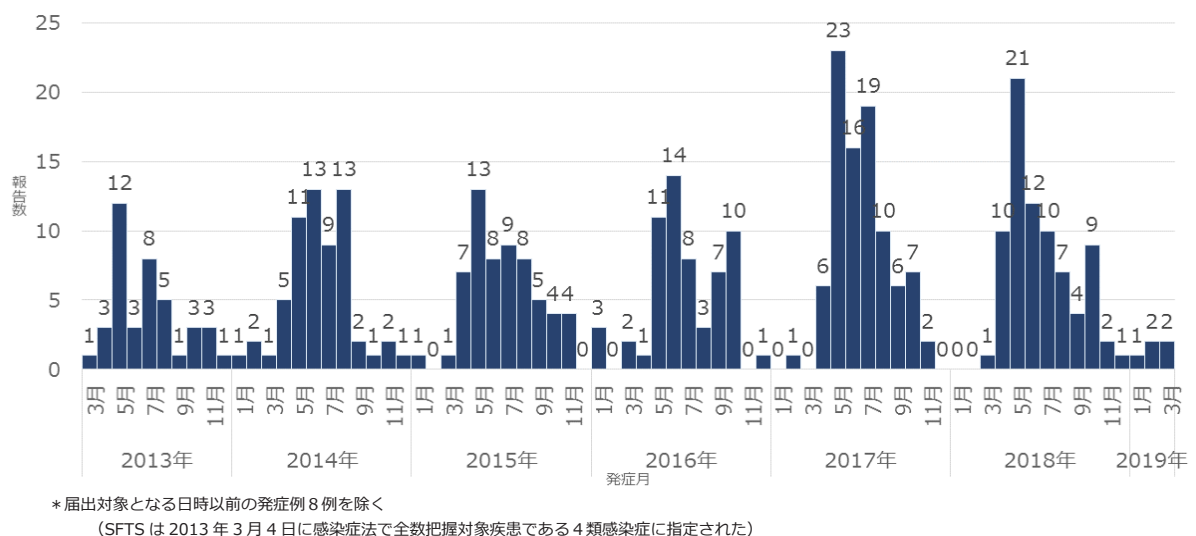
a) 2013 年 3 月以降に届けられた SFTS 症例の発症時期（n = 393, 2019 年 3 月 27 日現在）
