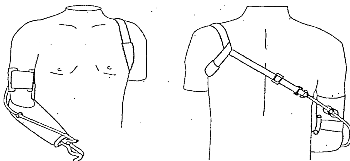
図-18 前腕義手用9字ハーネス式と 上腕カフの組合せ
