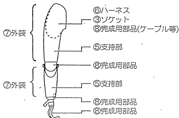
図－2 殻構造上腕義手の構成例
