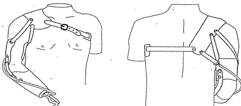
図-14 前腕義手用胸郭ベルトハーネス一式 (胸郭ベルトハーネス一式と上腕カフの組み合わせ)
