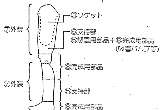
図－3 殻構造大腿義足の構成例
