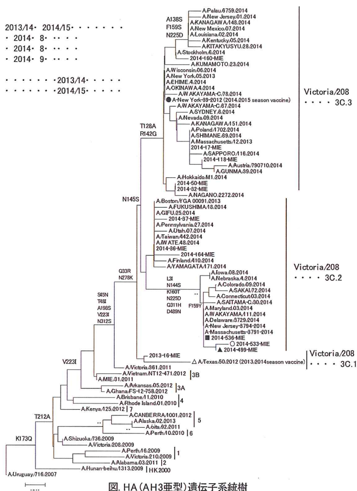
図. HA (AH3亜型) 遺伝子系統樹
