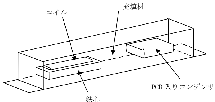
図－１ 蛍光灯用安定器の概略構造（例）
