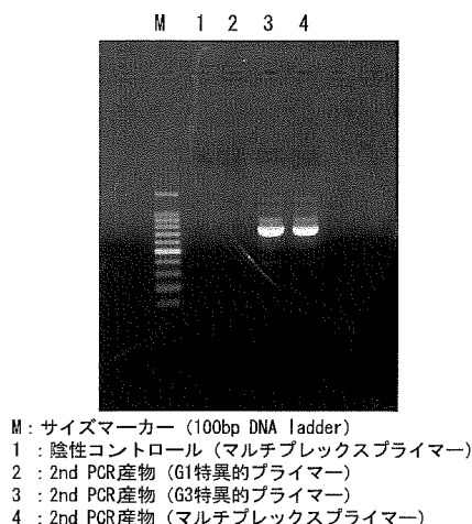
図1. アガロースゲル電気泳動によるマルチプレックスPCR法の増幅産物確認結果
