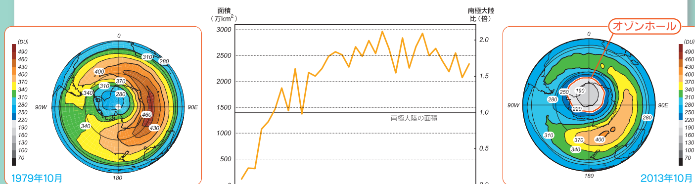
オゾンホールの年最大面積の経年変化（中央折れ線グラフ）と南半球の10月の月平均オゾン量の分布（左右図） データ提供：気象庁
