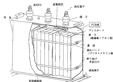
高圧コンデンサーの例
