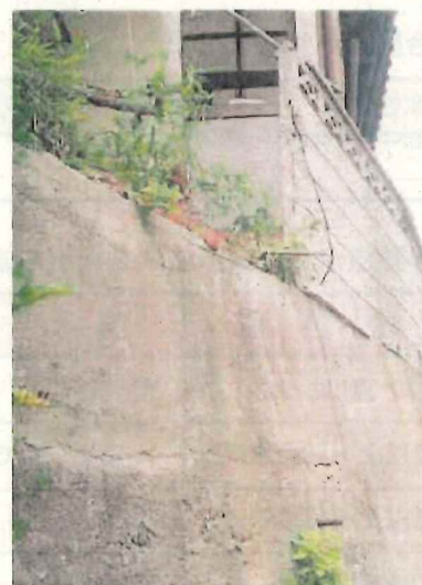
下部の擁壁と一体となるよう施工されず、落下したブロック塀
