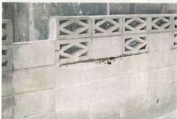
透かしブロックの直下の横筋が腐食し、地震で損傷した事例
