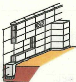
ブロック塀の仕組み
