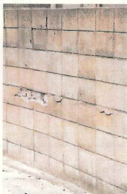
横筋が腐食・体積膨張し、ブロックを損傷している危険な塀
