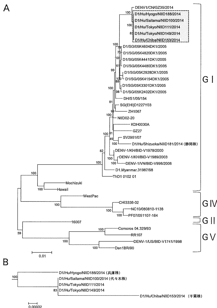
図. 2014年国内感染 Dengue 熱患者より同定された Dengue ウイルス 1 型全長ゲノムの系統樹解析 (文献 3 の図を改変)
