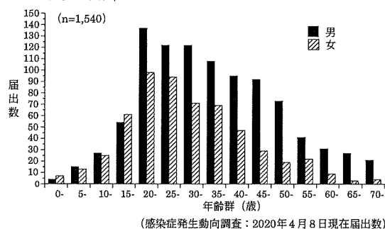
図2. デング熱・デング出血熱の輸入症例における性別年齢分布, 2015～2019年
