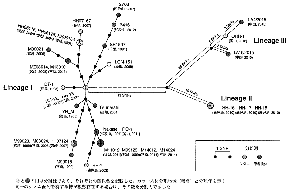
図2. 国内および中国で分離された33株の日本紅斑熱リケッチアの全ゲノム配列から推定される系統関係
