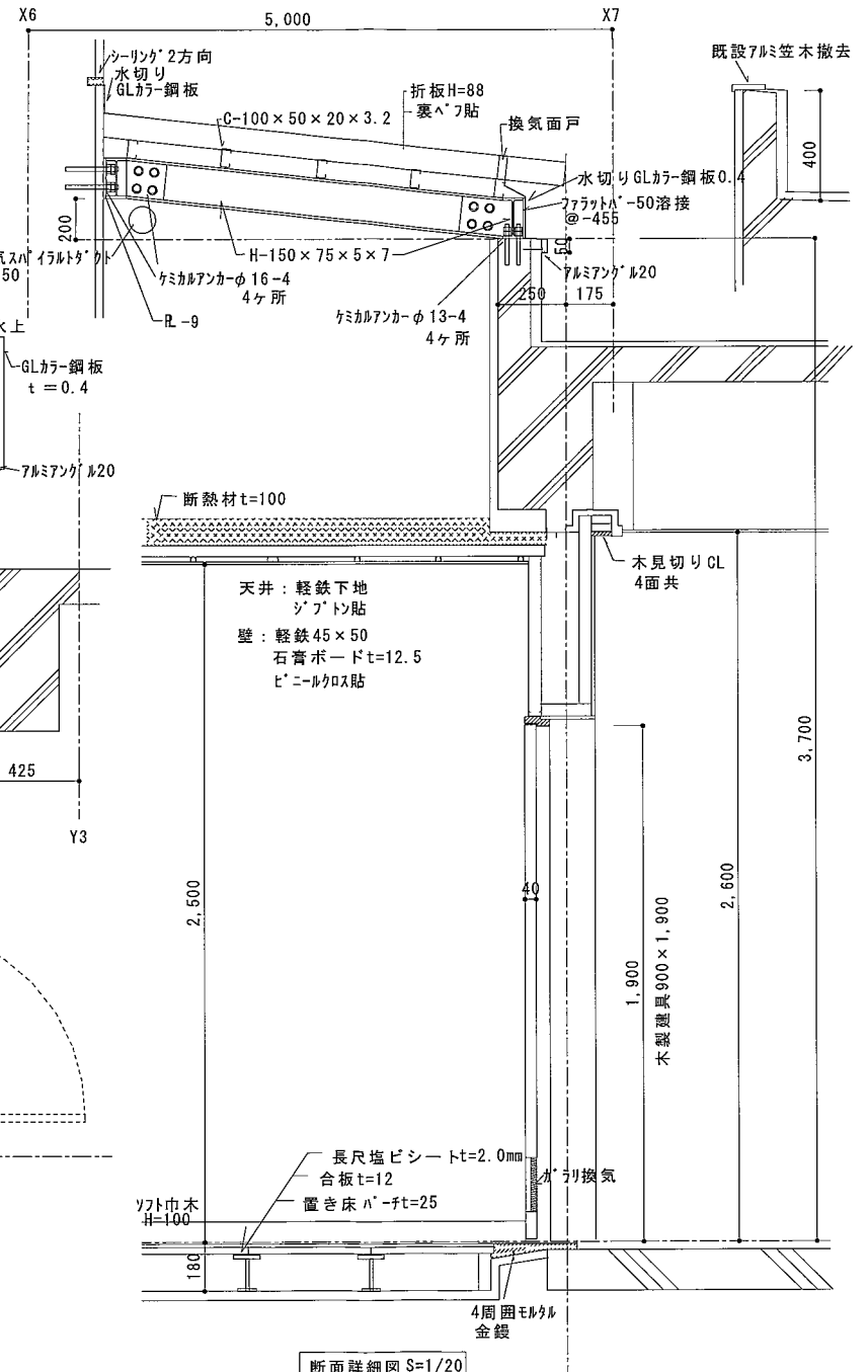
断面詳細図 S=1/20
