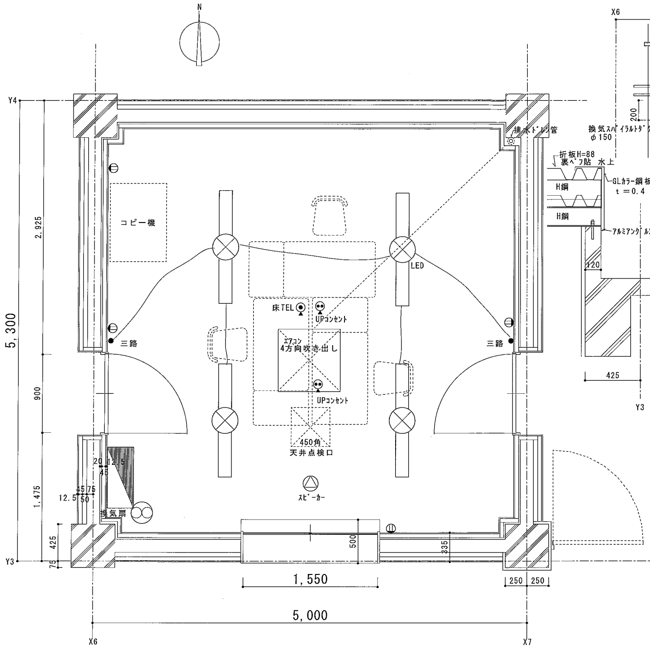
事務室平面図 S=1/30
